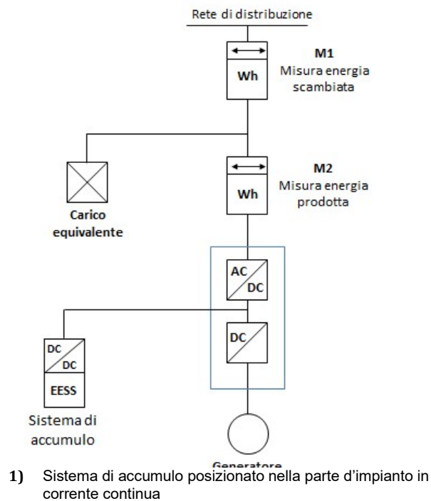
Figura 1: Schemi d'impianto realizzabili con FIM-HY-X.X-SE-A-1PH
